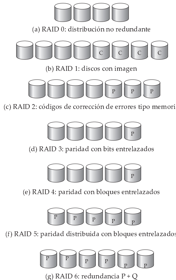
Figura 11.3 Niveles de RAID.
